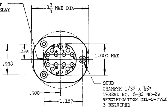
VIEW A-A
