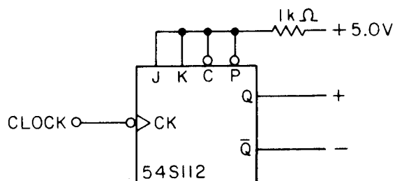
Flip flop input circuit.
